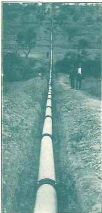
CONDUCCIÓN DE AGUAS EN CERVERA (Lérida) 1055 metros longitud - 250 m/m diámetro - 10 atmósferas
