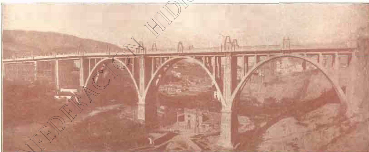
Viaducto de hormigón armado, de 250 metros de longitud, en Alzoy.
