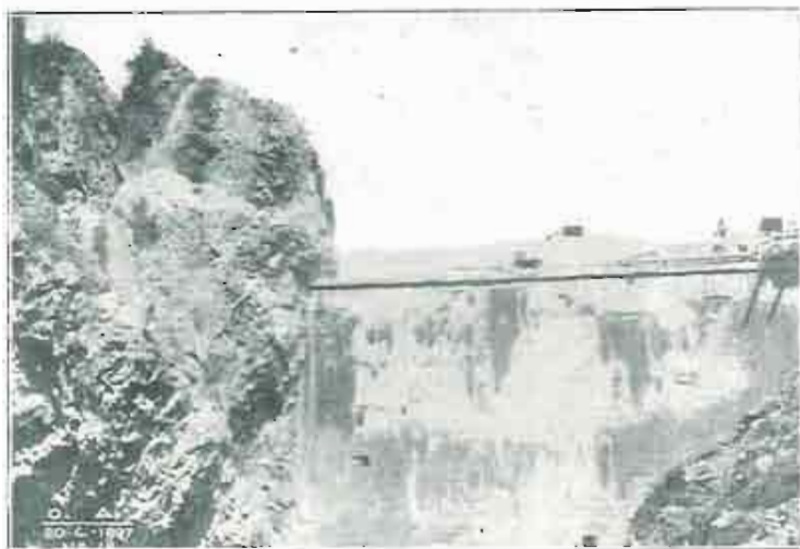
Estado de las obras de recrecimiento de la presa en 20 de Abril de 1927.
