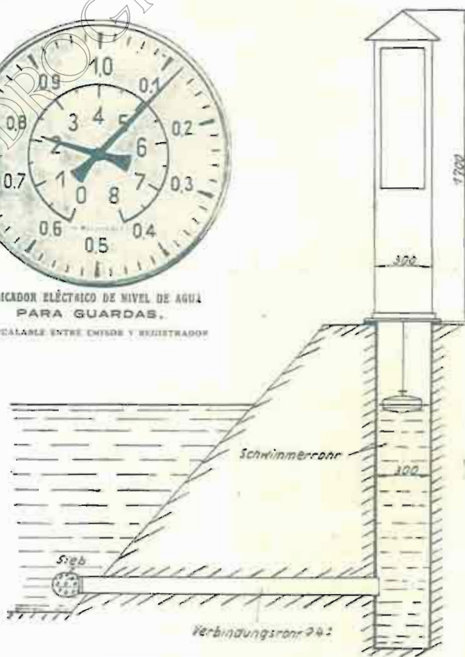
LIMNÍGRAFO «FUESS»
