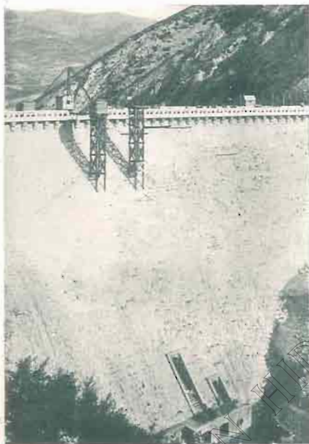
Figura 1.ª PANTANO DE SANTA MARÍA DE BELSUÉ. Vista parcial del paramento exterior de la presa.
