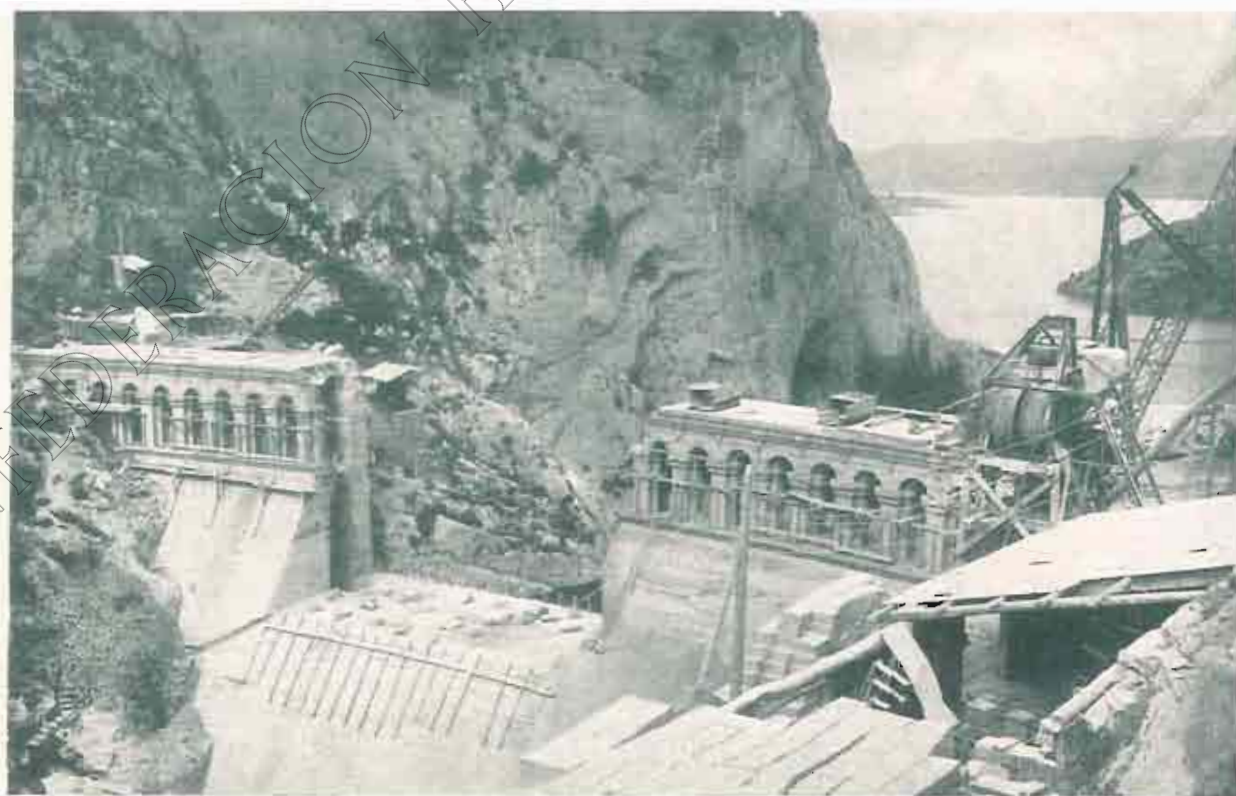
CORONACIÓN DE LA PIERA DEL PANTANO DE BARASONA. AL FONDO, EL EMBALSE (agosto 1930)
