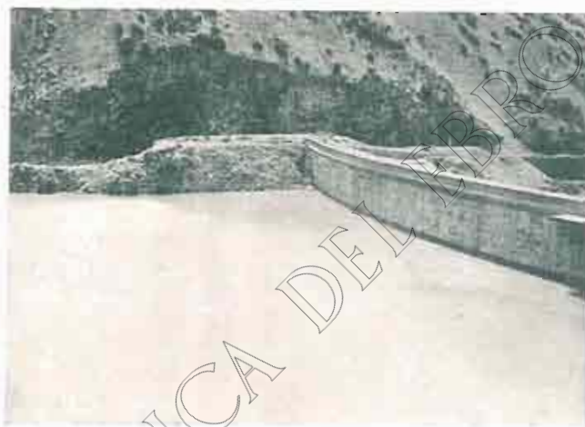
Figura 2.ª VISTA PARCIAL DE LA PRESA Y DEL ALIVIADERO. Máximo embalse, 1.º de julio de 1930: 6.800.000 m 3 . Altura del agua, 34 m.
