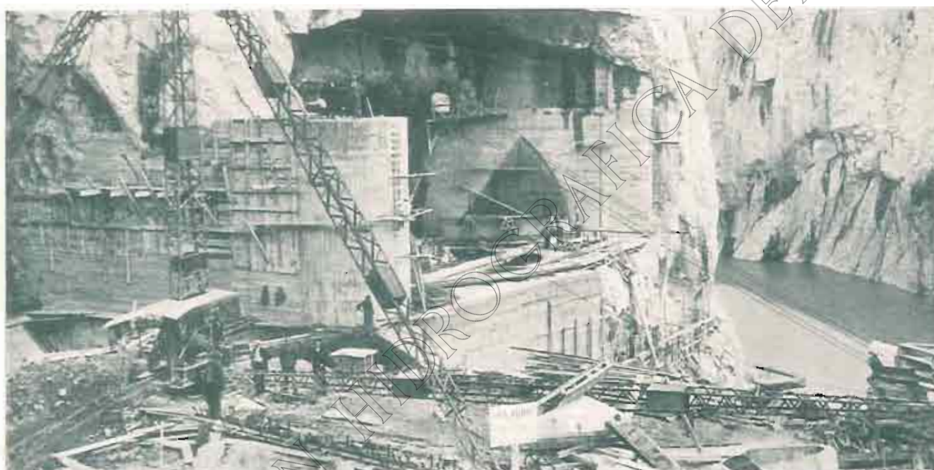
EMBOCADURAS DEL ALIVIADERO DE SUPERFICIE. INSTALACIÓN DE LAS ALZAS AUTOMÁTICAS (junio 1931)
