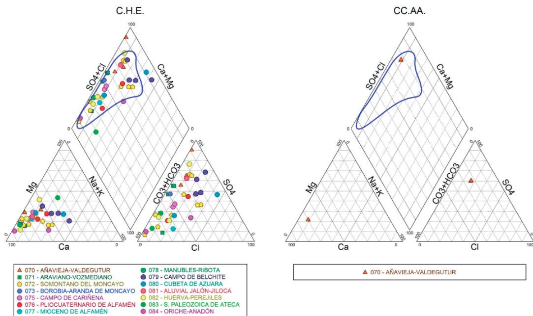
FIGURA 5.1.8 DIAGRAMA DE PIPER DEL DOMINIO CENTRAL IBÉRICO (IZDA. RBAS, DCHA. CCAA)
