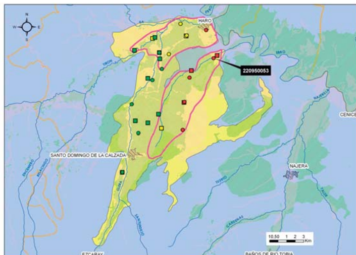
FIGURA 5.2.10 CONCENTRACIÓN PROMEDIO DE NO 3 - DURANTE EL AÑO 2011 EN LOS PUNTOS DE CONTROL DE LA MASA DE AGUA SUBTERRÁNEA "ALUVIAL DEL OJA"
