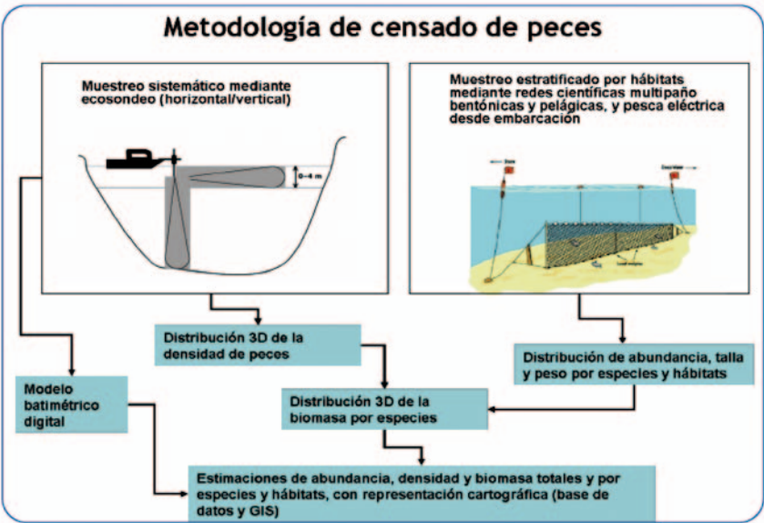
■ FIGURA 3.2 ESQUEMA DEL MÉTODO DE CENSADO DE POBLACIONES ÍCTICAS EN UN EMBALSE
